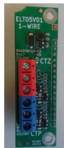
Rys.12. Kolejność zacisków ELT05 opisana kolorami: brązowy, biały, zielony
