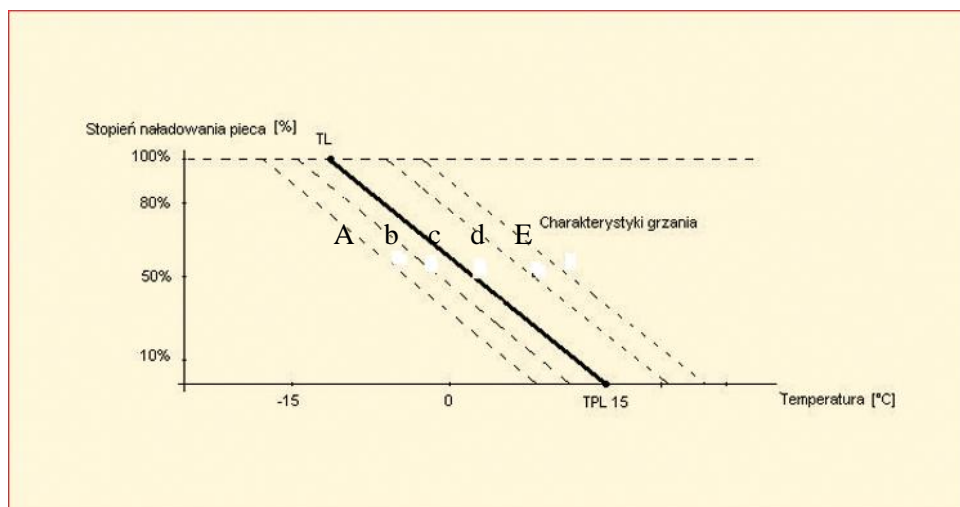
Rys.1 Przykład wykresu krzywej ładowania ogrzewacza (linia wyłuszczonej) oraz możliwości zmian poziomów ładowania w zależności od ustawień przez Użytkownika oczekiwanego komfortu (funkcji) grzania.
